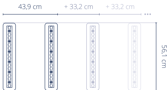
Wandmodule 56 | Wall Module 56
