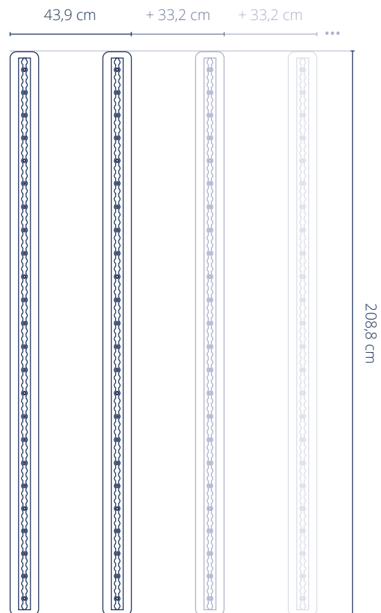
Wandmodule 209 | Wall Module 209
