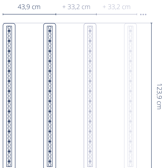
Wandmodule 124 | Wall Module 124
